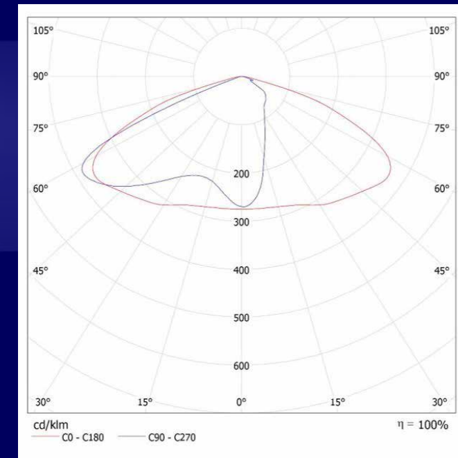
Distribution photométrique de STRETON LED 150W.
